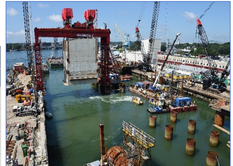
PNSY DD 1 Monolith Install
